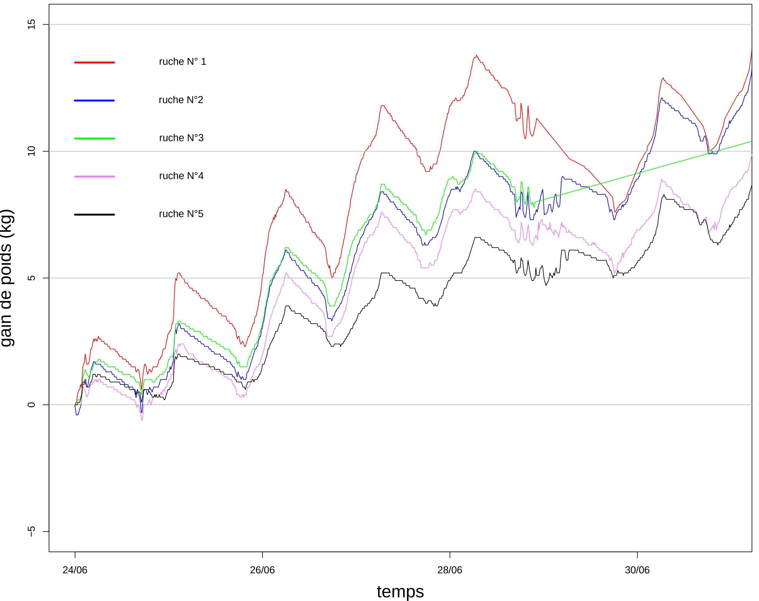
VD24 – Montagnac (courbe de gain de poids, corrigée du poids des hausses rajoutées)
