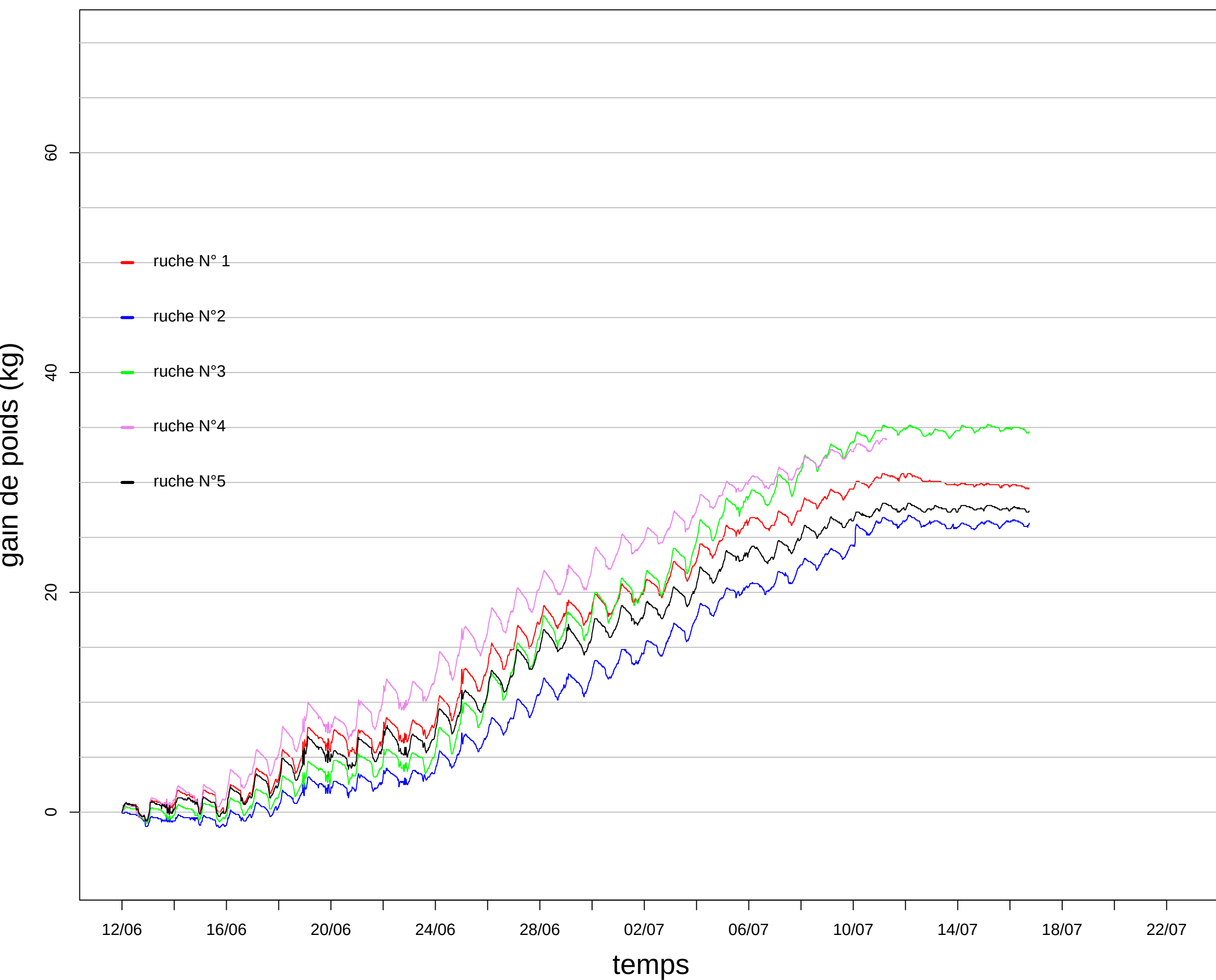
DA24 – Valaurie (courbe de gain de poids, corrigée du poids des hausses rajoutées)
